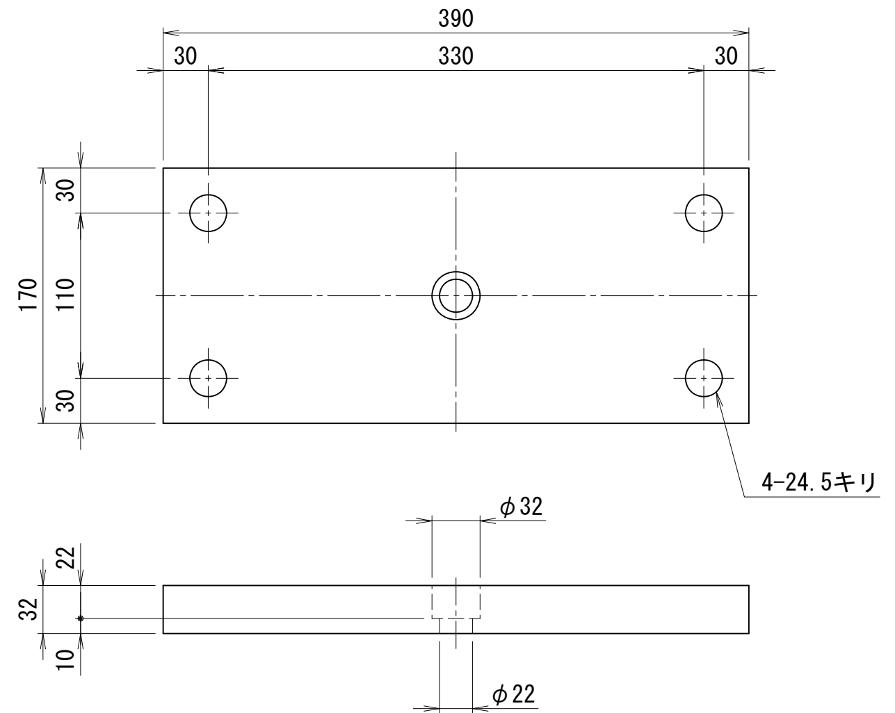
2000kN用ヘッド取付けプレート 約16kg
