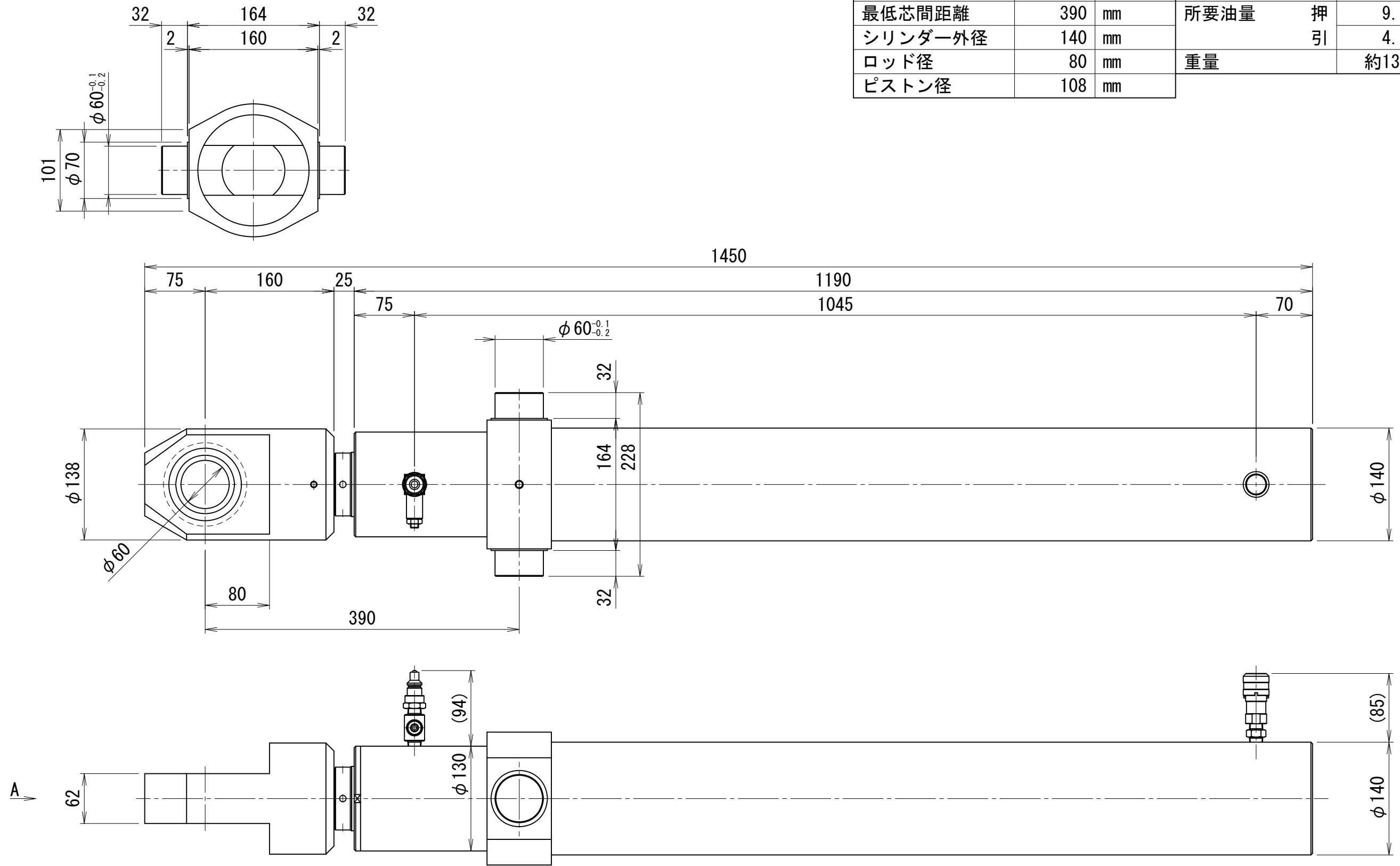
A矢示図
