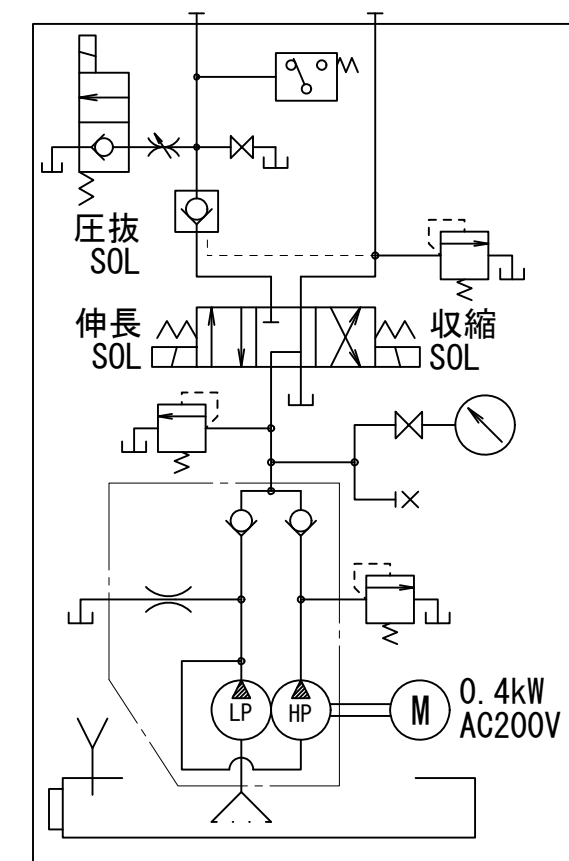
油圧回路図
