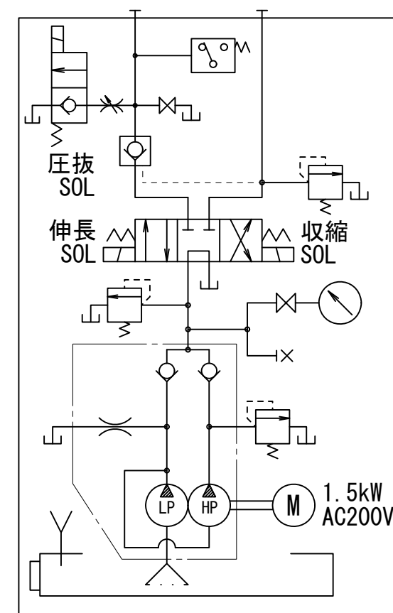
油圧回路図
