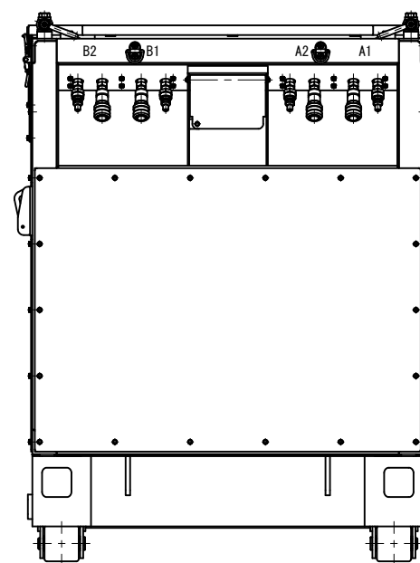
A矢示図
