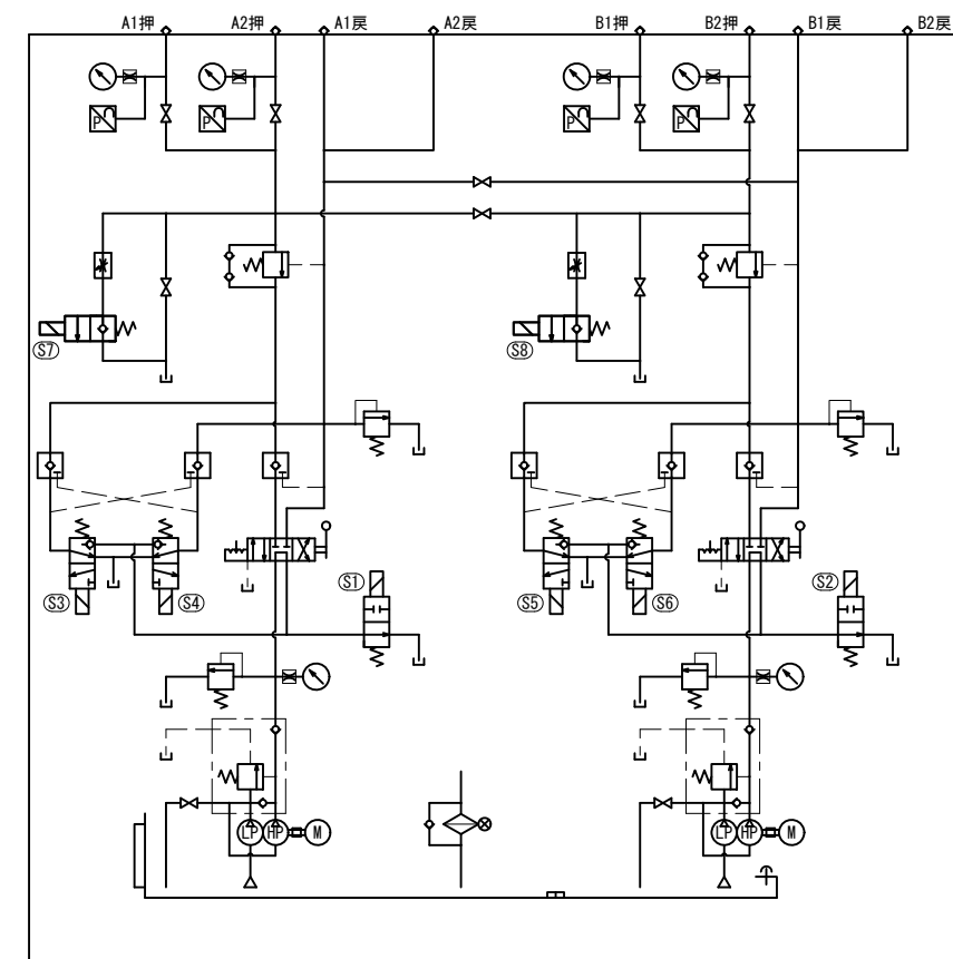
油圧回路図
