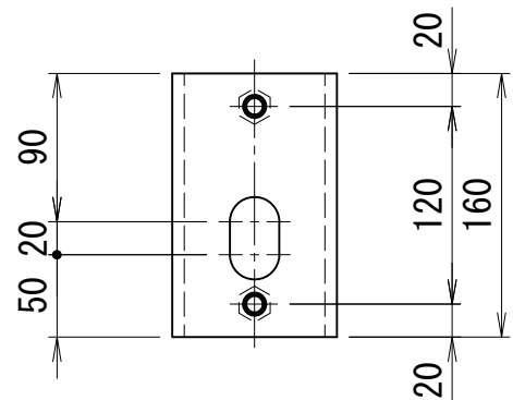
ブラケット詳細
