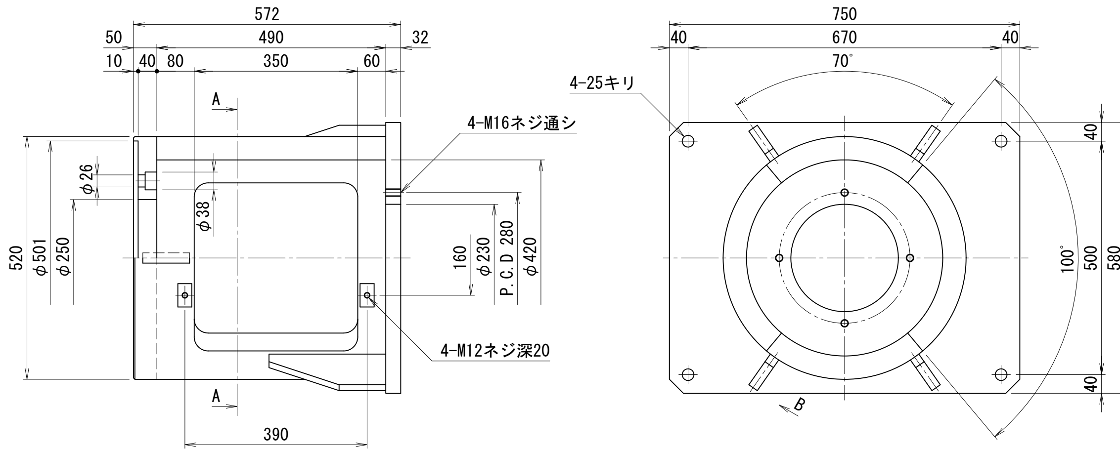
A-A断面図
