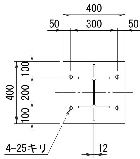
A-A断面図
