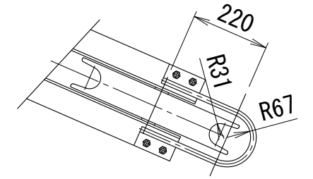
B矢示図
