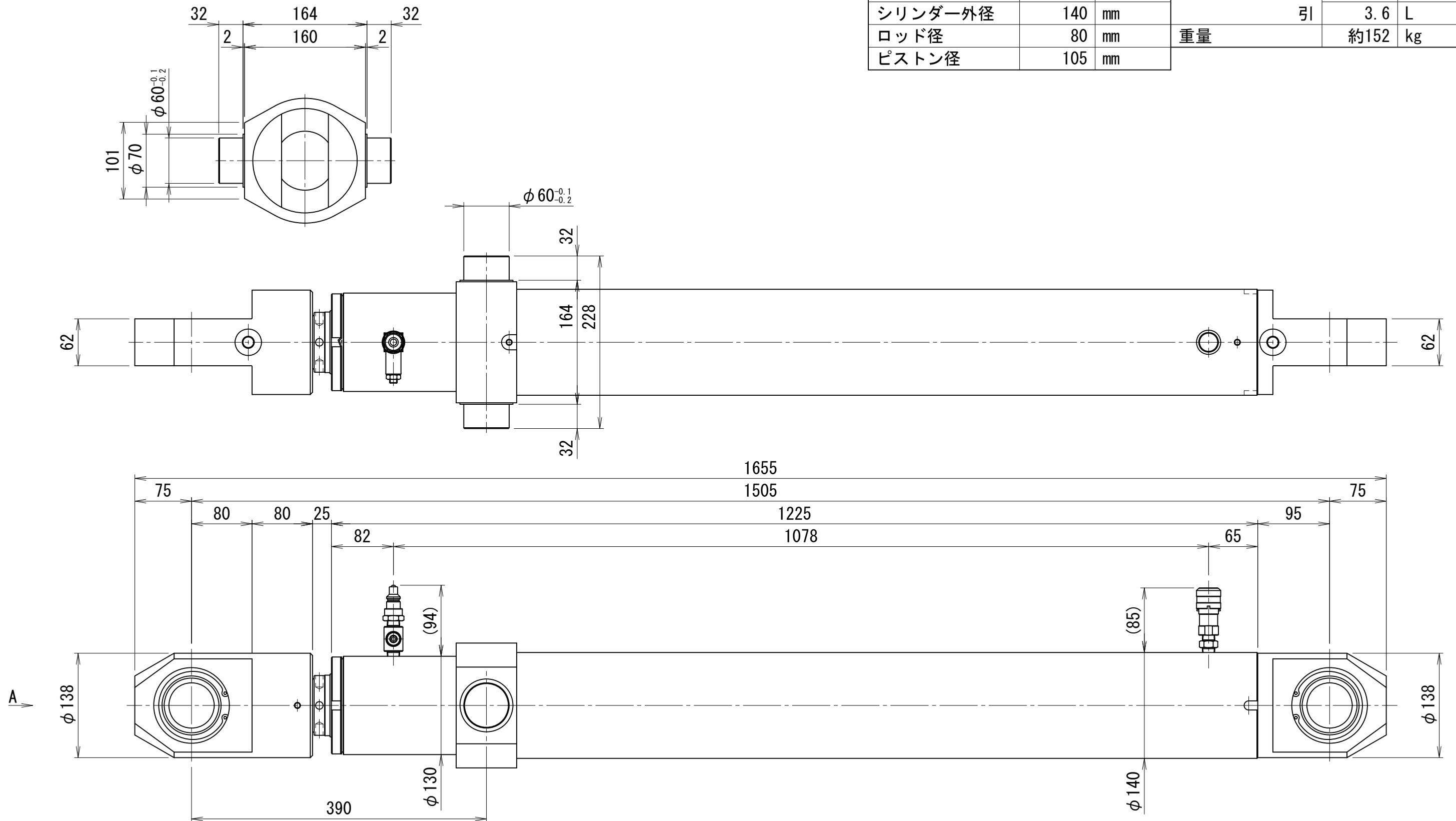
A矢示図
