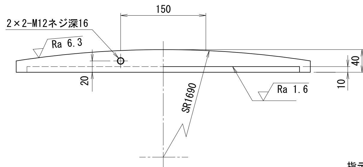
A-A断面図
