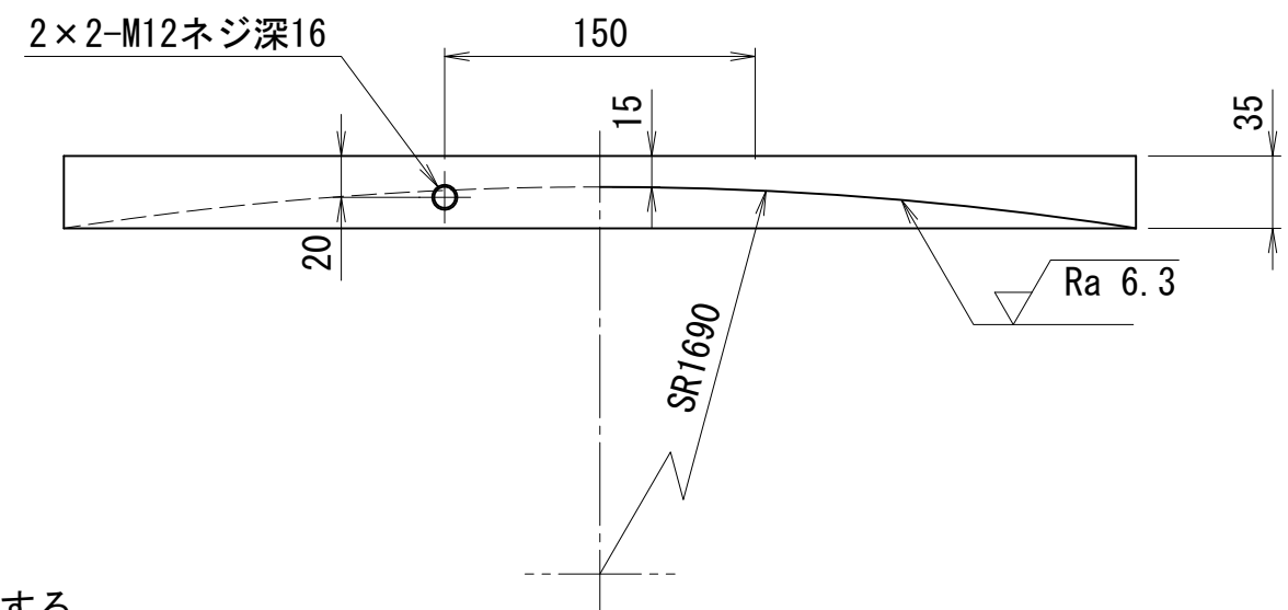
A-A断面図
