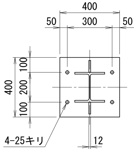
A-A断面図
