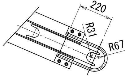
B矢示図
