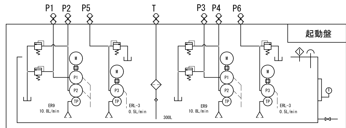
油圧回路図
