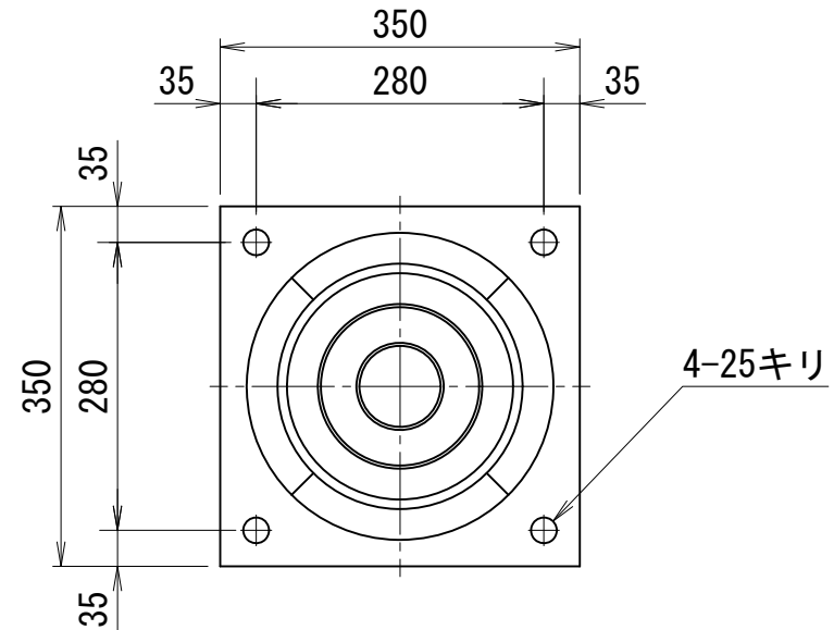
A矢示図
