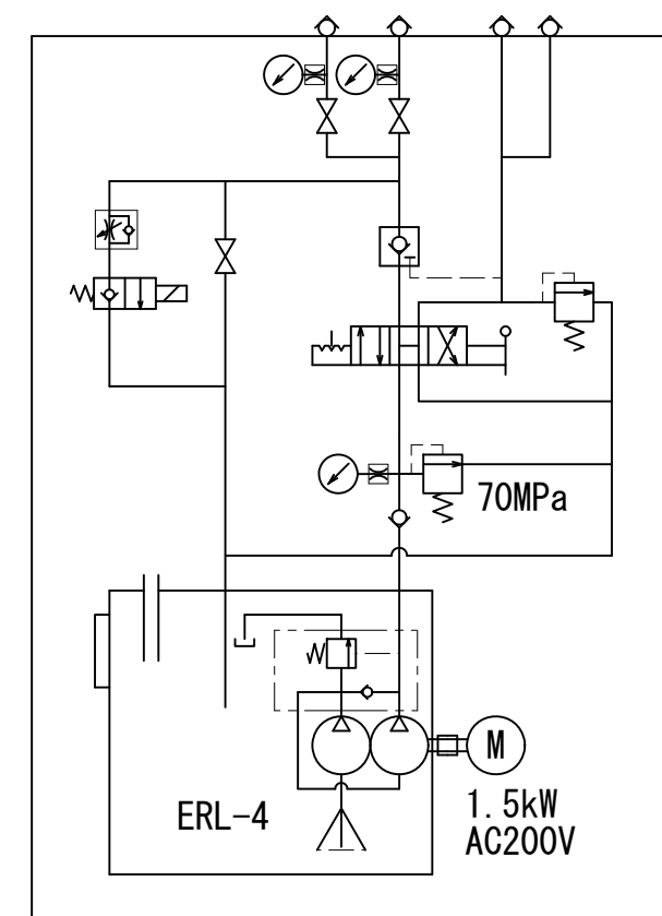
油圧回路図
