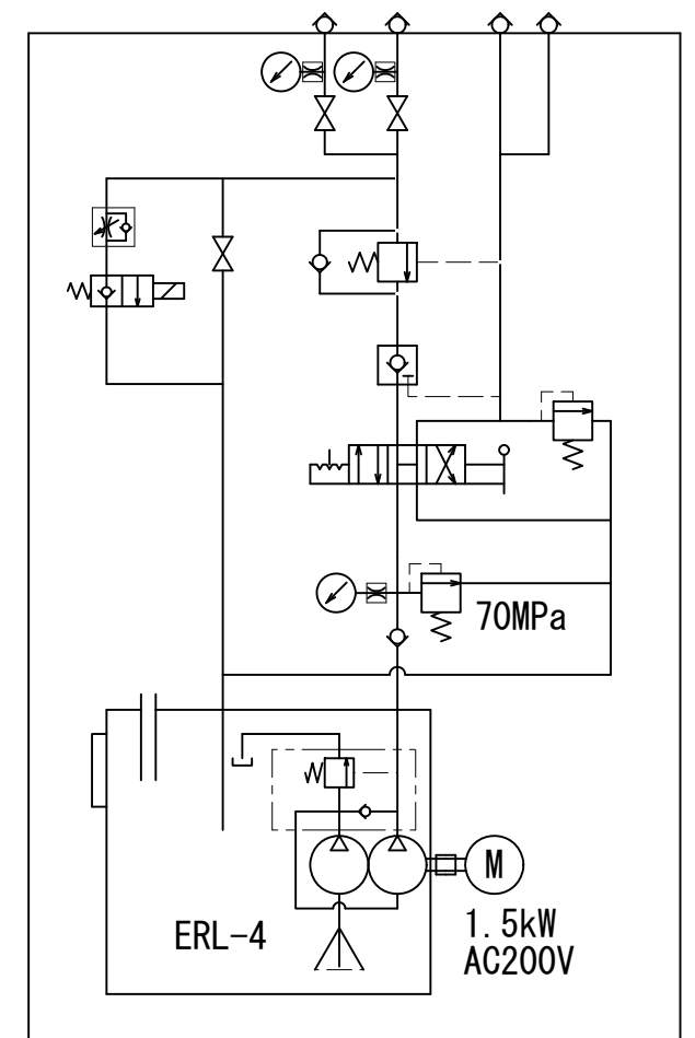
油圧回路図
