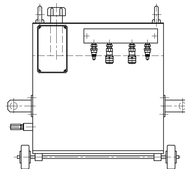
A矢示図
