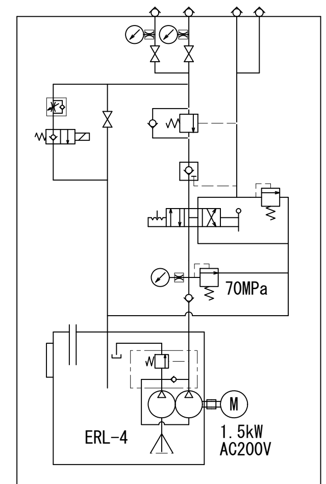
油圧回路図
