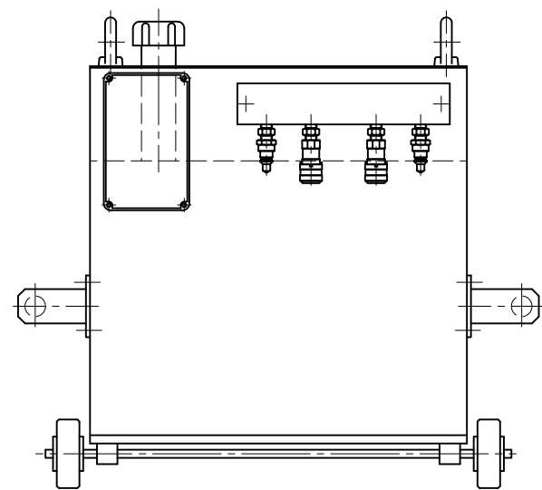
A矢示図
