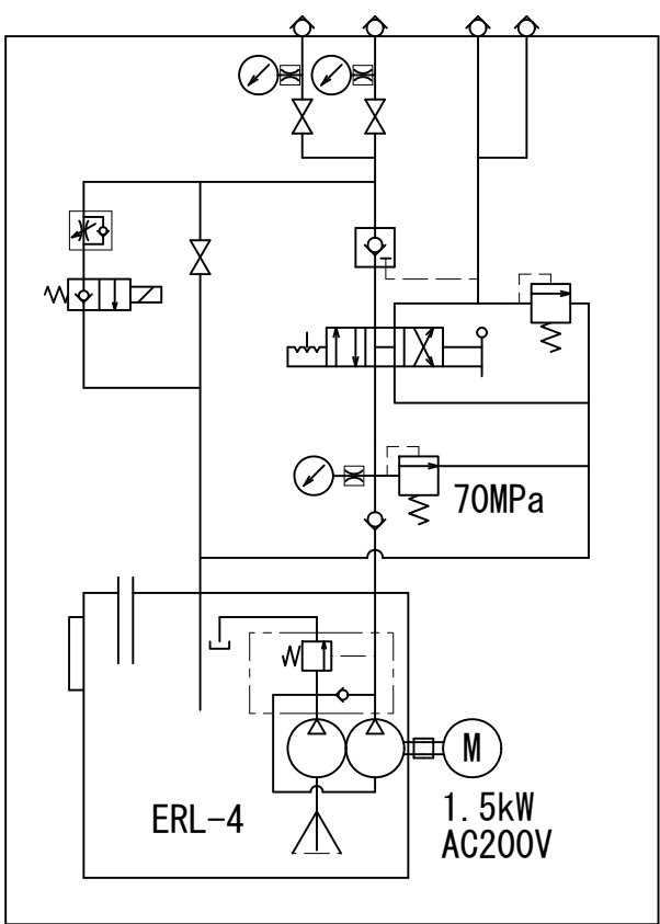
油圧回路図
