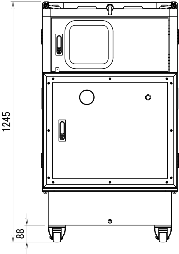
オイルパン取付け状態
