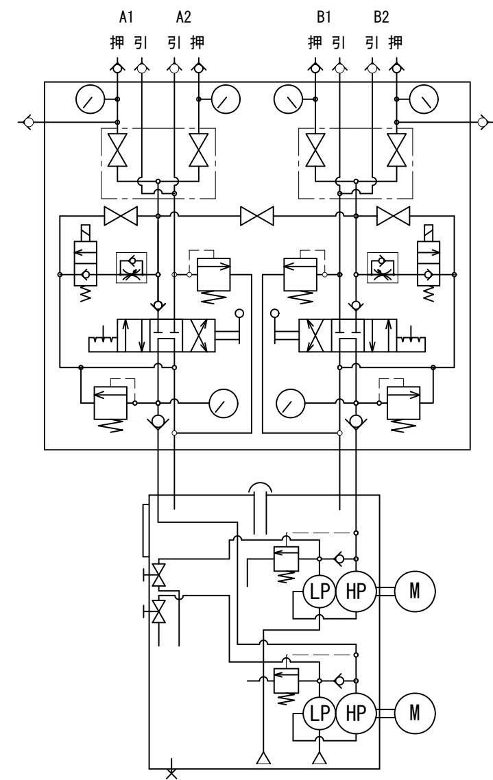
油圧回路図
