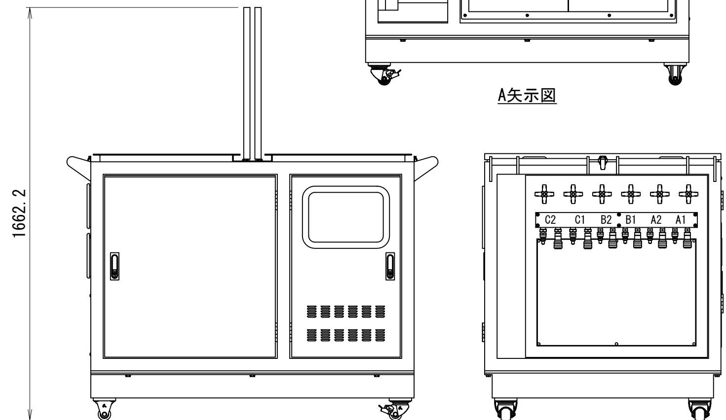
上部点検扉解放状態
