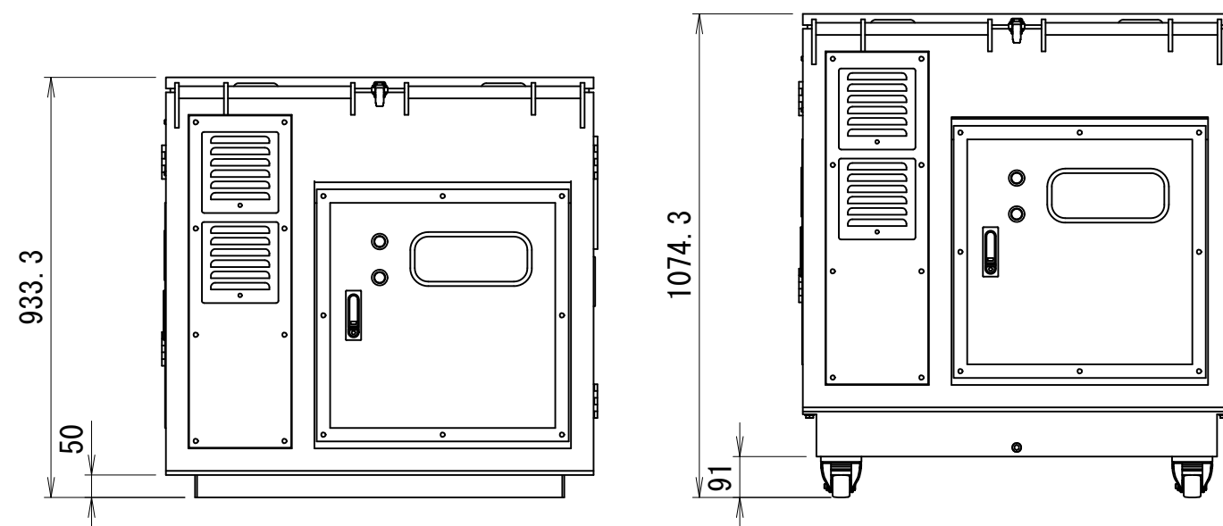
オイルパン取外し状態
