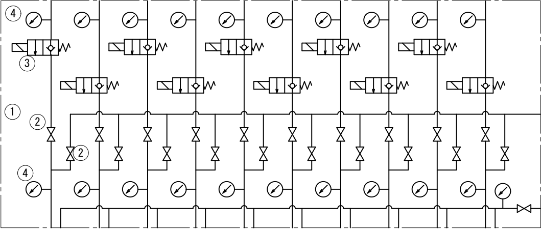
回路図
