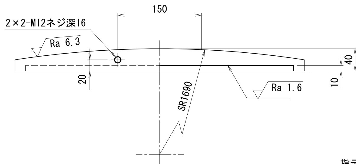
A-A断面図
