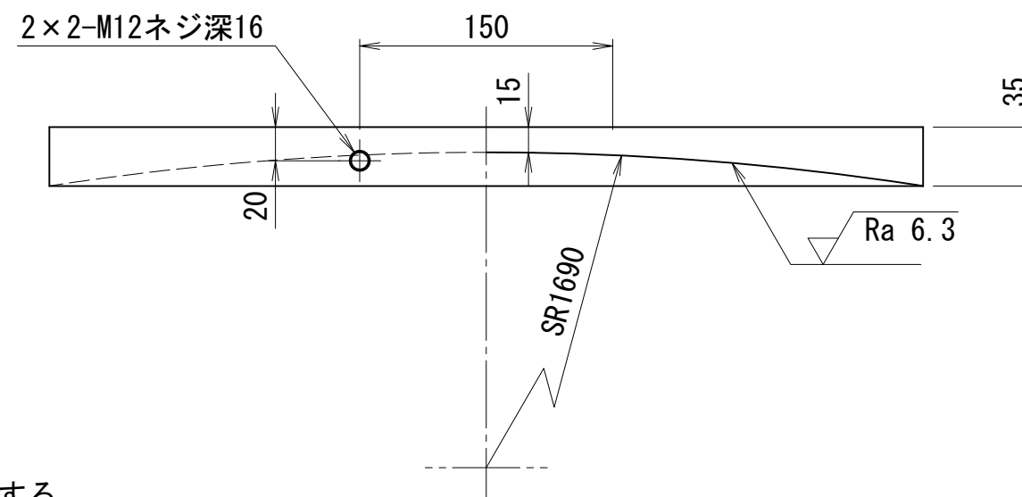
A-A断面図
