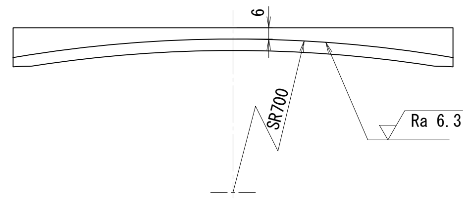
A-A断面図
