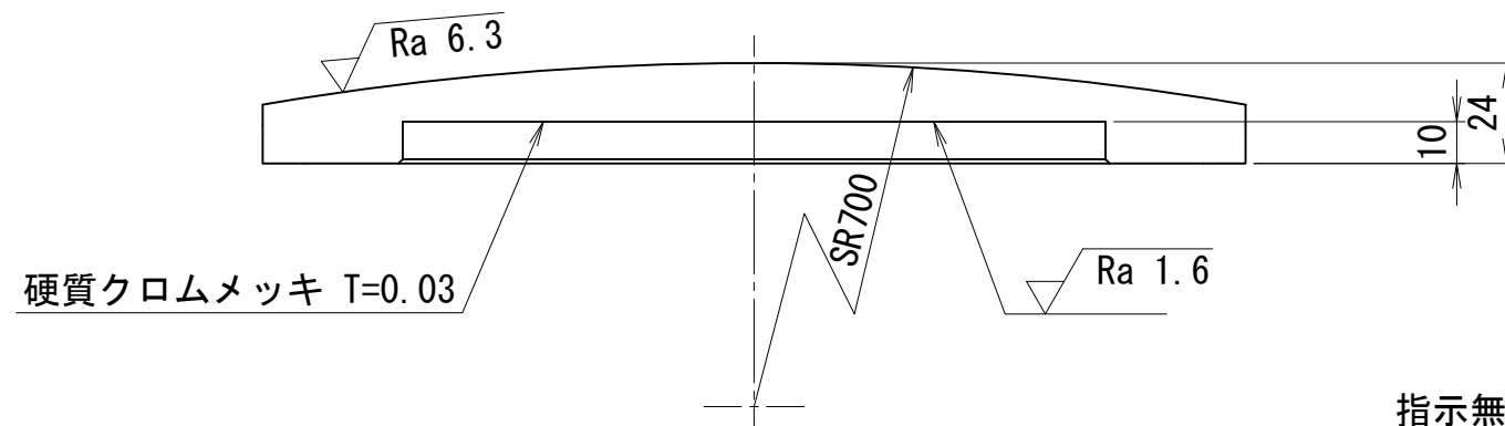
A-A断面図
