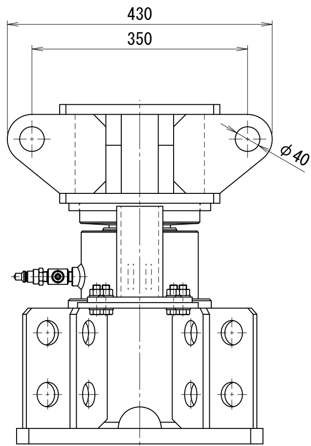
A矢示図
