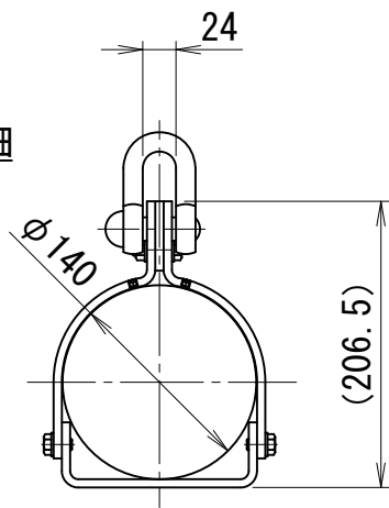
吊金具詳細
