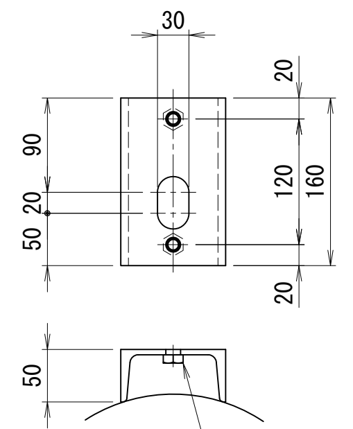
ブラケット詳細
