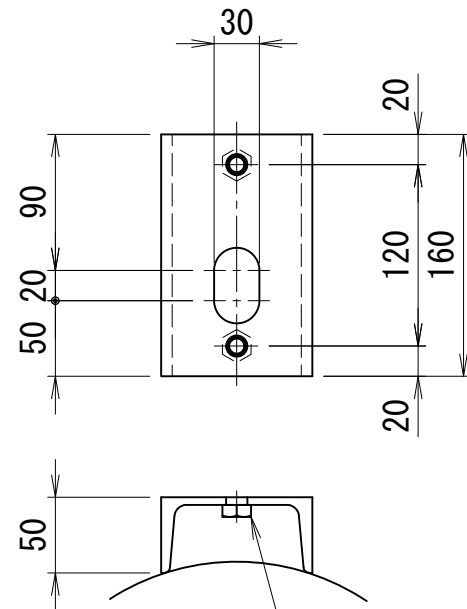
ブラケット詳細
