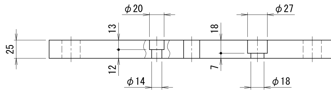
A-A断面図
