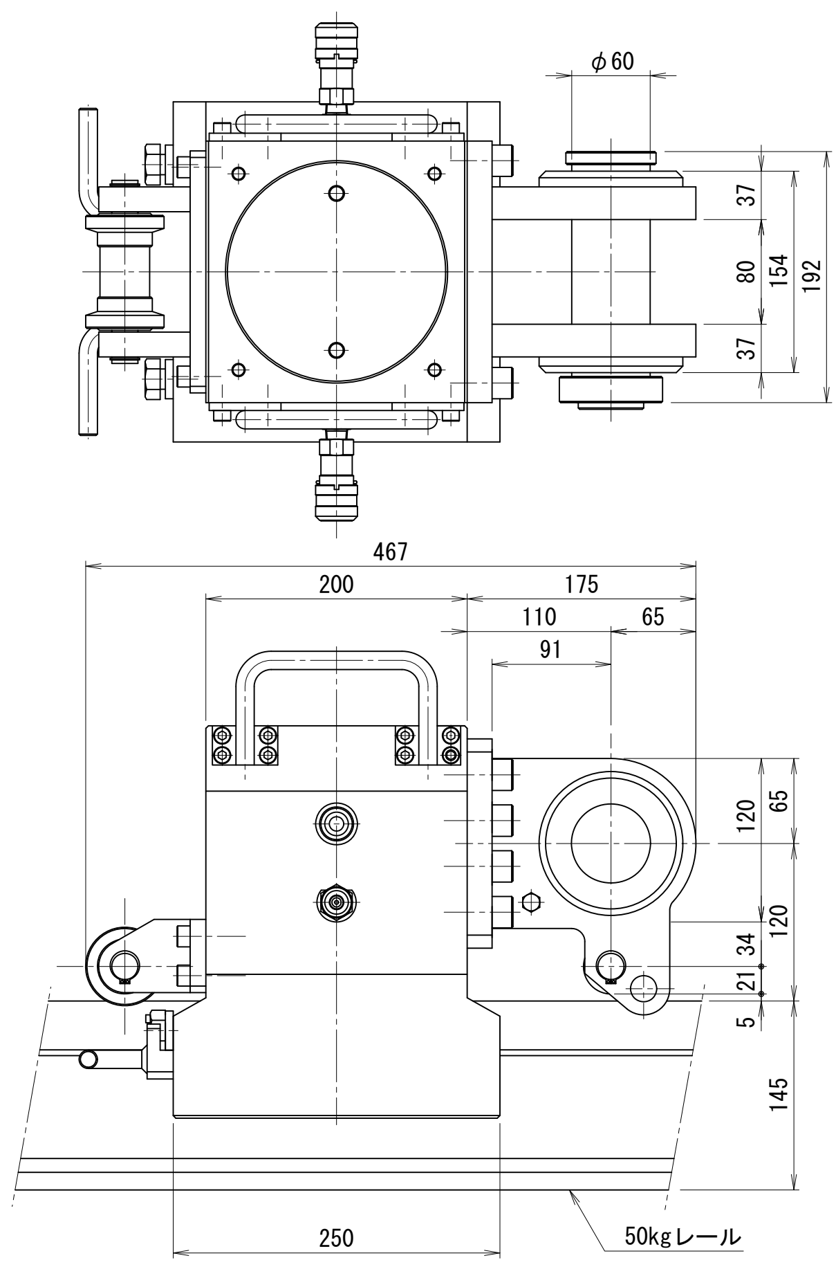
50kg レール用クランプ装置 TYPE-4
