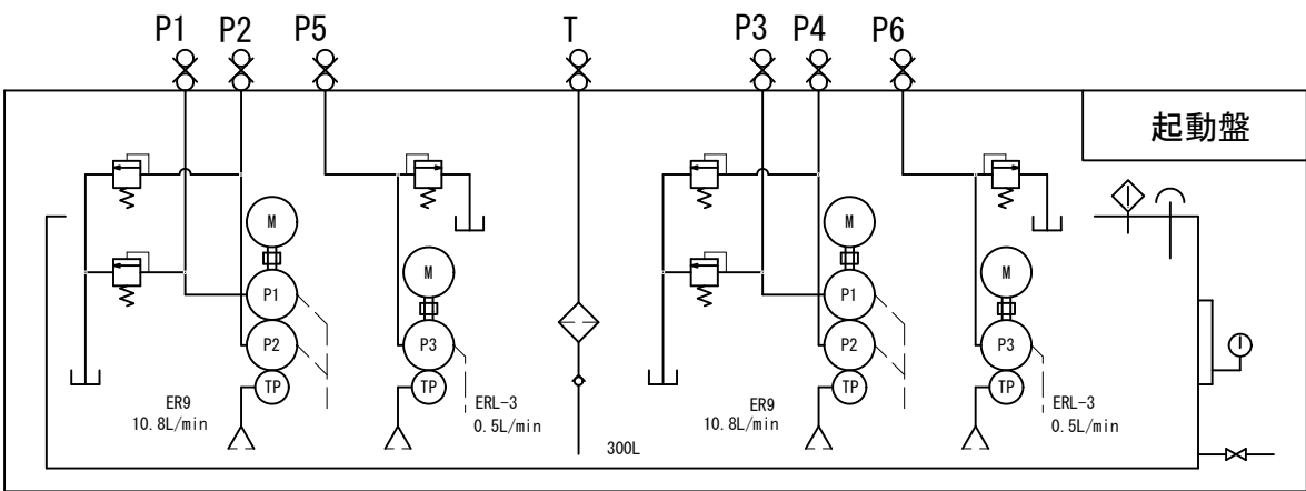
油圧回路図
